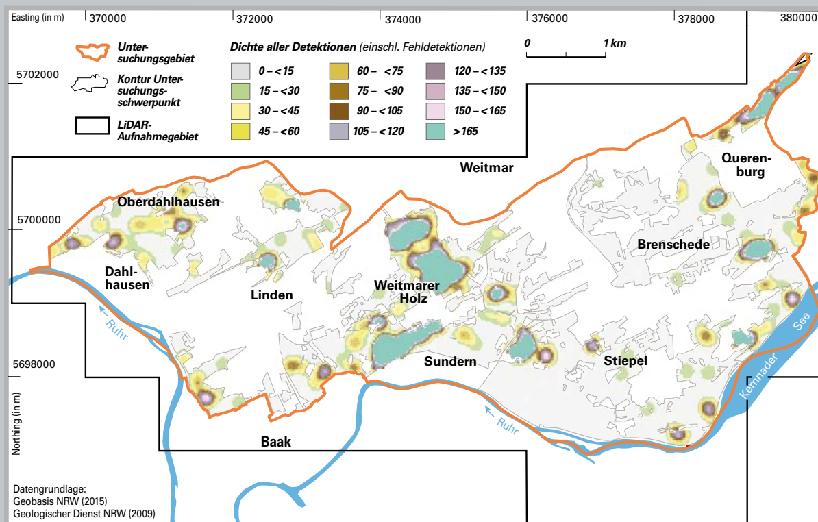
Abb. 26: Punktdichtemessung (kernel-density) aller klassifizierten Detektionen
