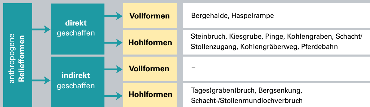
Abb. 1: Gliederung anthropogener, altbergbauspezifischer Reliefformen
