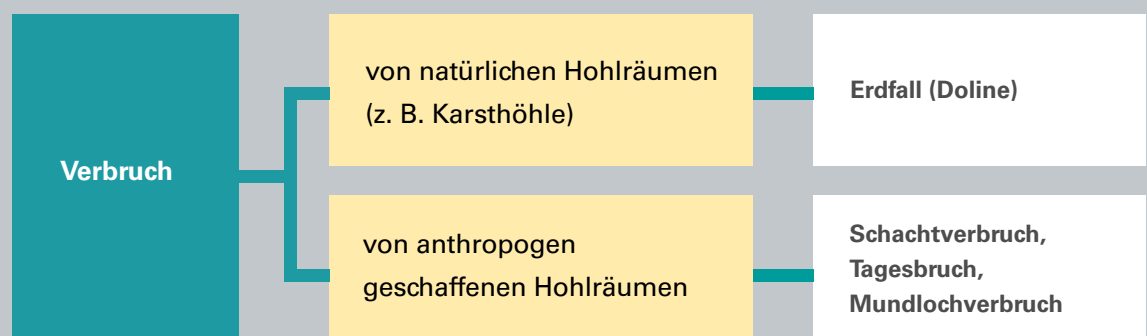
Abb. 7: Definition des Begriffs „Verbruch“ (verändert nach MEIER, G. & MEIER, J. 2007: 92)
