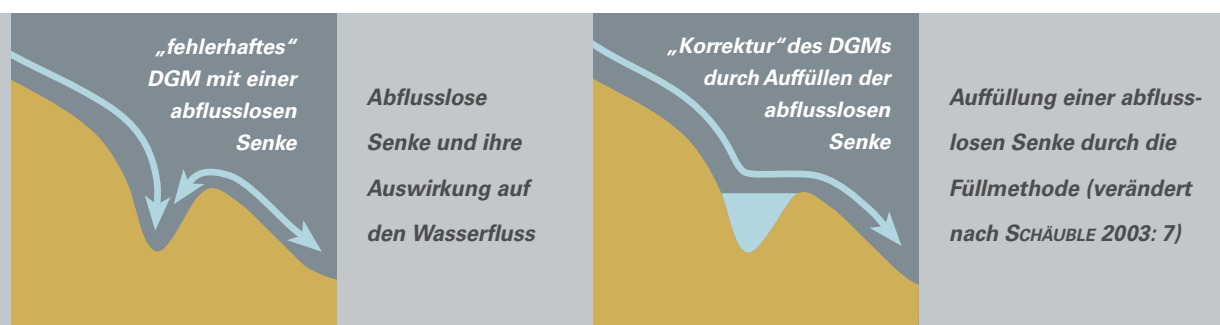
Abb. 16: Detektion abflussloser Senken im DGM mit der Füllmethode
