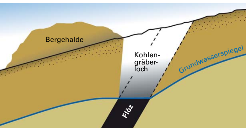
Abb. 6: Der Ausbiss eines Kohlenflözes und die Grundwasserproblematik der frühen Kohlengräberei (verändert nach BADER & RÖTTGER 1987: 22)
