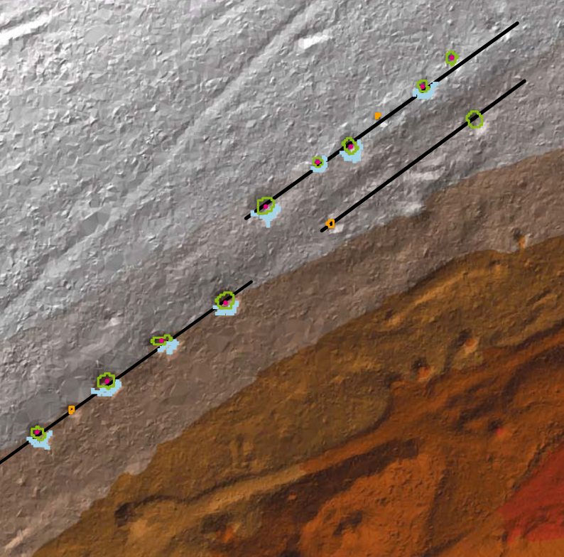
Abb. 23: Auswahl perschnurartig in NE-Richtung aufgereihter Hohl- und Vollformen: Die räumliche Anordnung und die hangabwärts gelegenen 0-Akkumulationsflächen ließen eine eindeutige Klassifizierung als Kohlengräberlöcher, die Teil eines Pingenzuges sind, zu.
