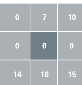
b) In den höchstgelegenen Bereichen gibt es keine Abflussakkumulation.
